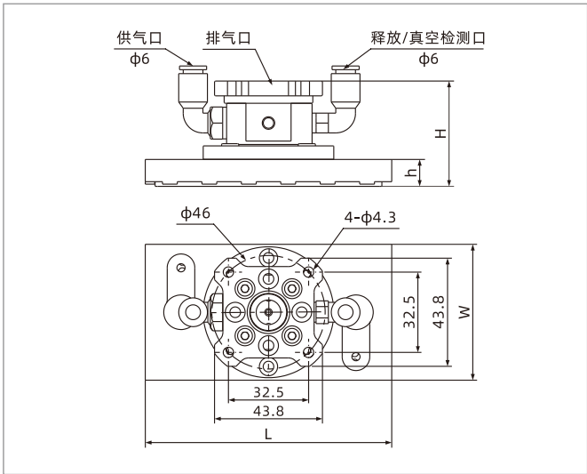
SLW□PK-M10I-F1
